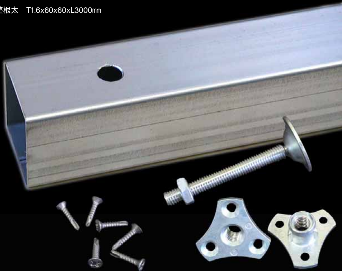
鋼製レベル調整根太(ZAM®使用) 詳細図
