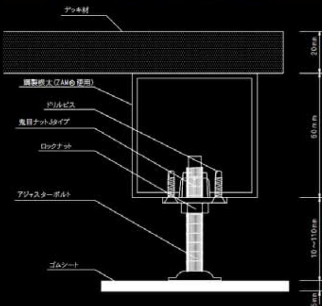
鋼製レベル調整根太(ZAM®使用) 詳細図
