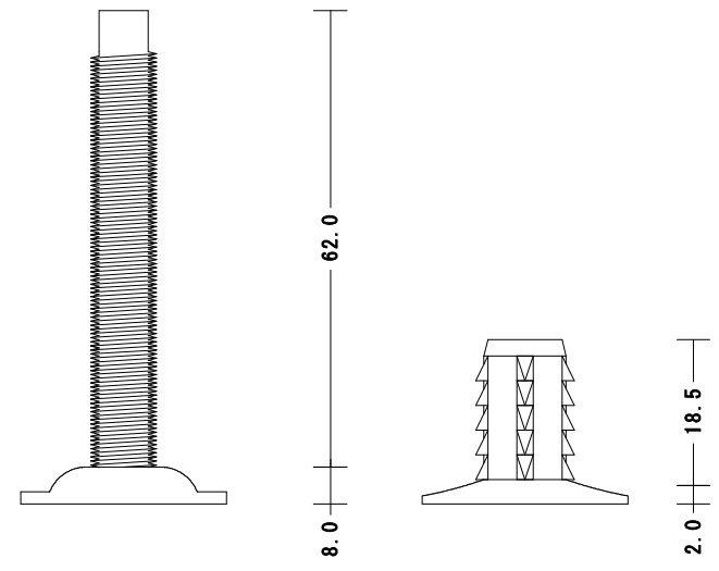
アジャスター M8 x L70mm
